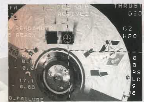
Graphische Darstellung der Station bei der Annäherung des ATV. Der dicke blaue Punkt in der Bildmitte ist das Heck des russischen Swesda-Moduls, wo sich das Kopplungsaggregat befindet. Rechts ein Fernsehbild der Endphase.
